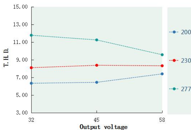
T.H.D. VS Output voltage(DL-200H-58A/S-MAL)
