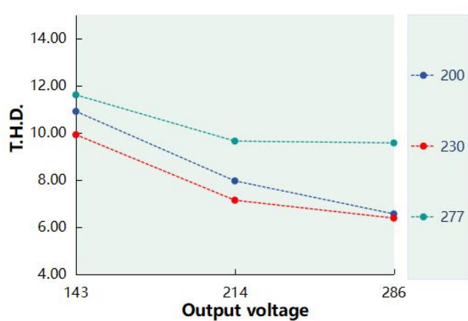
T.H.D. VS Output voltage(DL-200H-286A/S-MAL)
