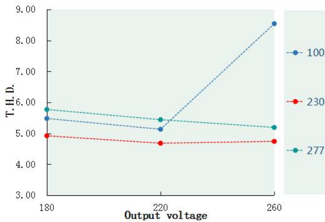
T.H.D. VS Output voltage (DL-240Z-260A/S/X -PXG)
