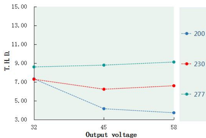
T.H.D. VS Output voltage(DL-50H-MAL)
